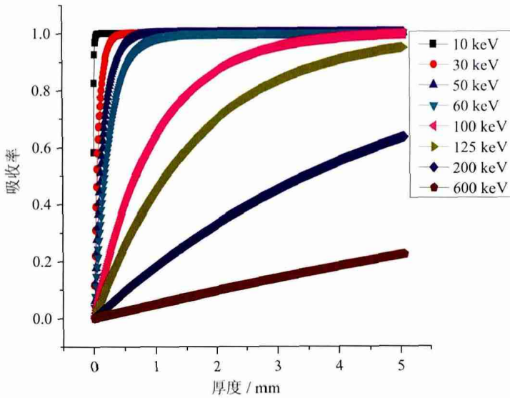
图1 不同能量的X射线在不同厚度的CdZnTe中的吸收率
